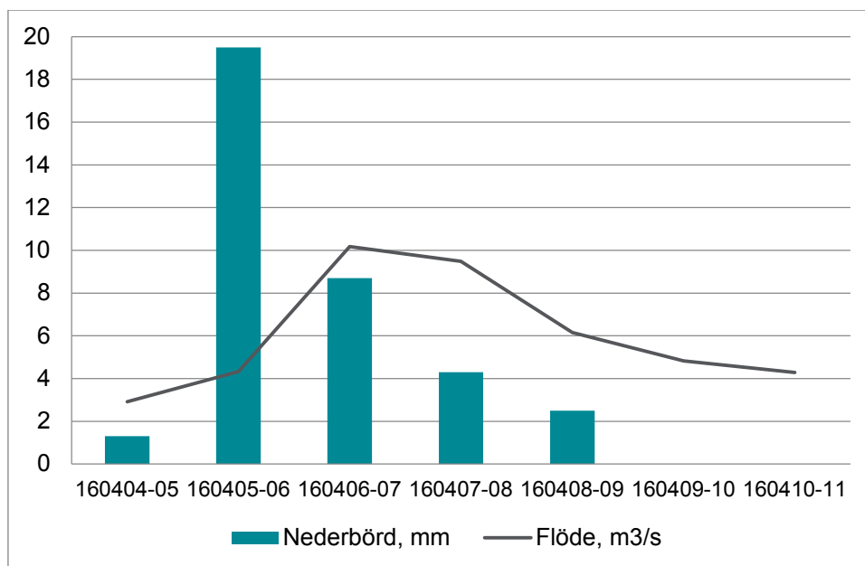
Figur 6. Variation i flöde och nederbörds mängd under provtagningsveckan.
