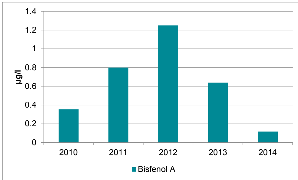
Figur 5. Halten bisfenol A i utgående vatten från Ryaverket (Screeningdatabasen, ivl.se).
