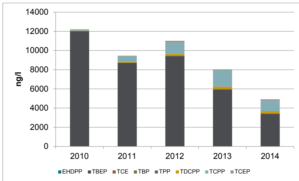
Figur 2. Halten organofosfater i utgående vatten från Ryaverket för åren 2010 till 2014 (Screeningdatabasen, ivl.se).
