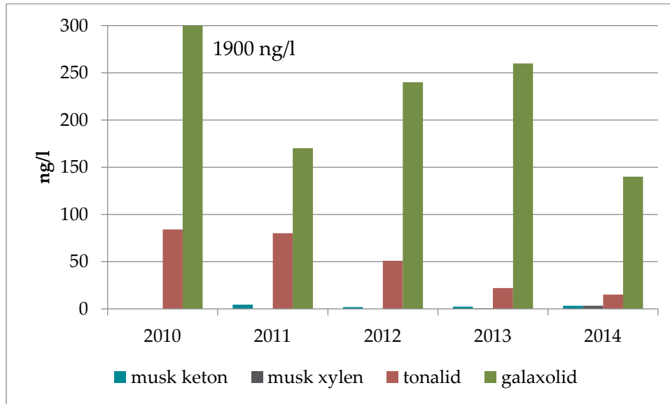
Figur 3. Halter av myskämnen i utgående vatten från Rya, 2010-2014 (Screeningdatabasen, ivl.se).
