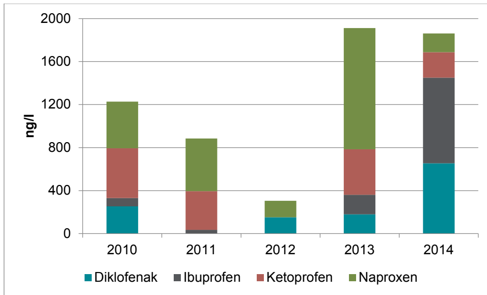
Figur 4. Halten NSAID's (ibuprofen, ketoprofen, naproxen och diklofenak) i utgående vatten från Ryaverket, 2010-2014 (Screeningdatabasen, ivl.se).
