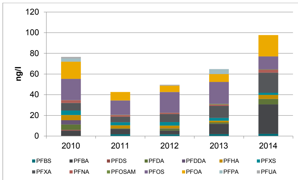
Figur 1. Koncentration av perfluorerade ämnen i utgående vatten från Ryaverket för åren 2010 till 2014 (Screeningdatabasen, ivl.se).
