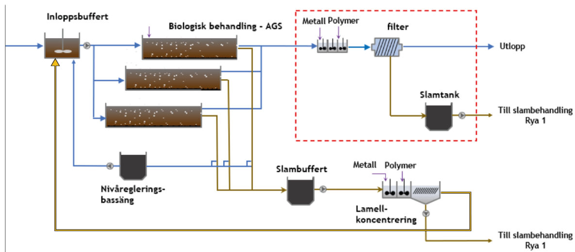
Figur 6-5 Schematiskt flödesschema över AGS-anläggningen på Rya 2. Streckad röd ruta innehåller tertiärbehandlingen (fällning och filtrering) på Rya 2. Slammet från tertiärbehandlingen (benämnt filter i figuren) kan även skickas till lamellkoncentrering.
